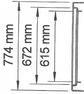
Schnitt Einstieg
